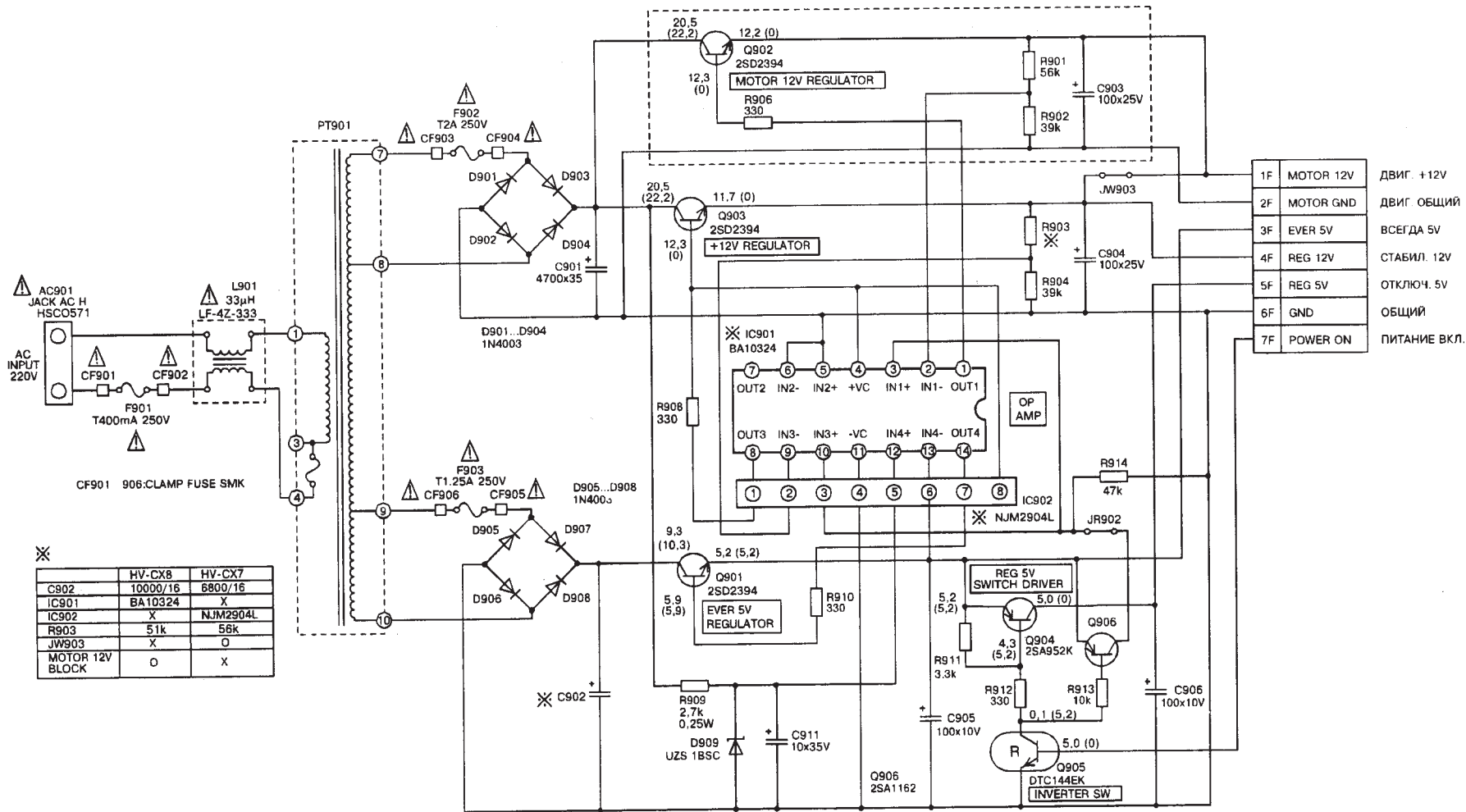
Рис. 2.6. Принципиальная схема источника питания видеоплейеров HV-CX7/CX8.
